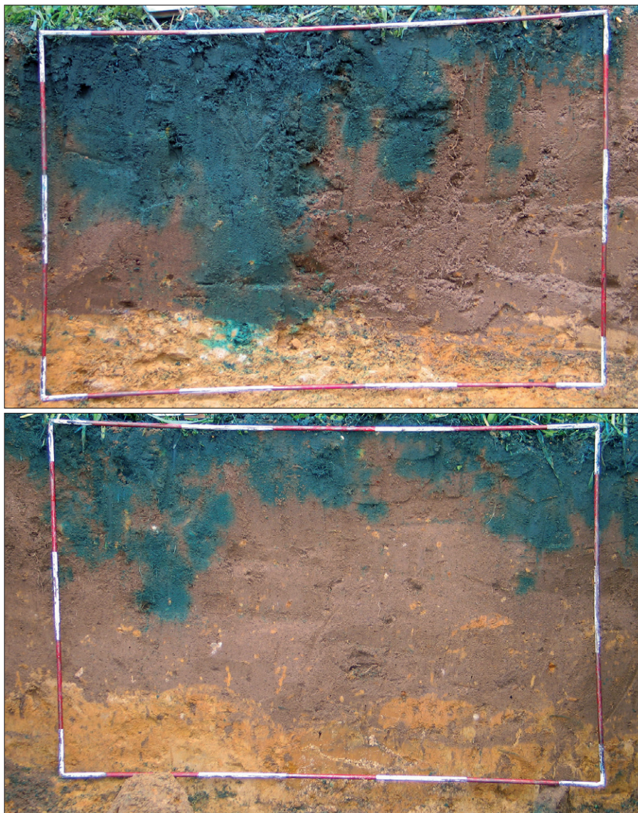
Obr. 7. Znázornění průniku vody do půdy po deseti měsících od kypření do různé hloubky: nahoře po kypření do hloubky 0,32 m; dole bez hlubšího kypření
