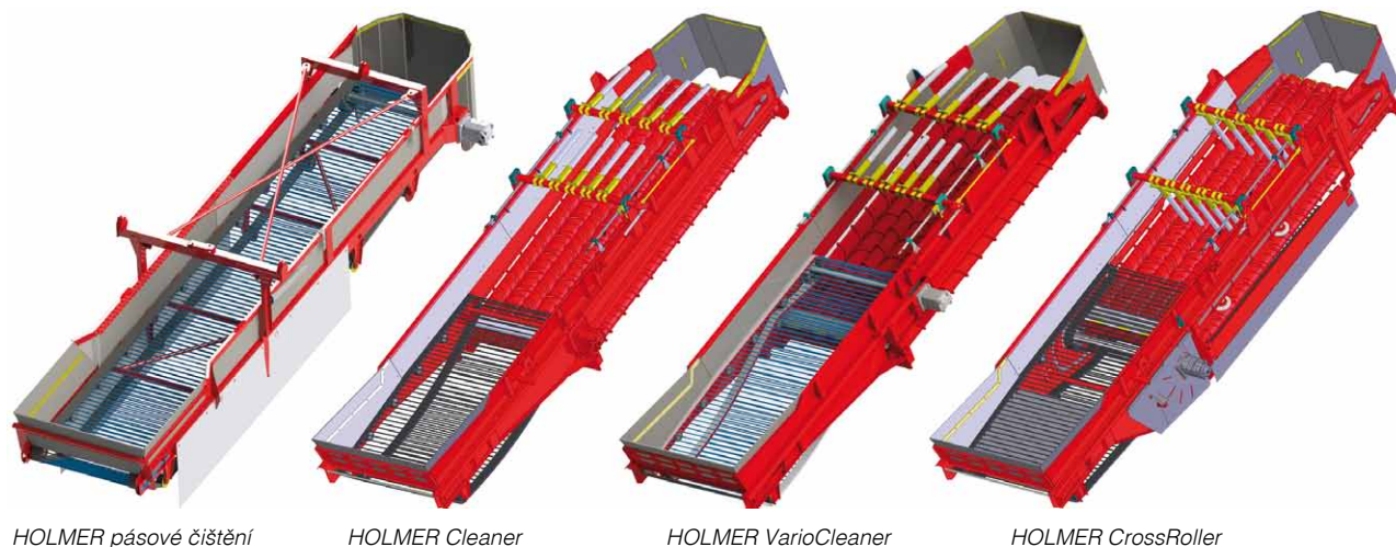
Obr. 1. Systémy dočištění u čistícího nakladače Terra Felis 2 eco
