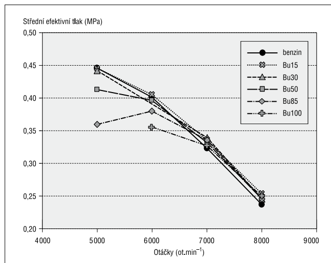
Obr. 2. Porovnání vnějších otáčkových charakteristik motoru bez úprav karburátoru
