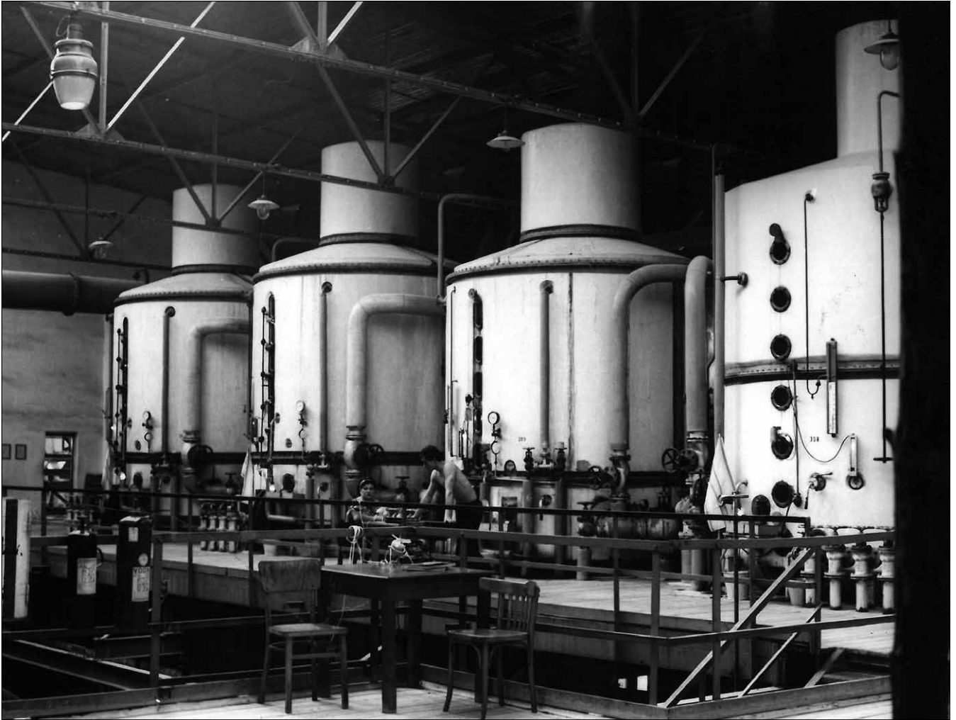
Obr. 8. Surovinové zrníče v novém cukrovaru (1968)
